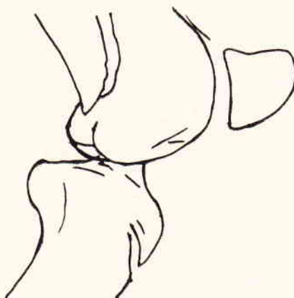
Ryc. 2. Szkic rentgenogramu
